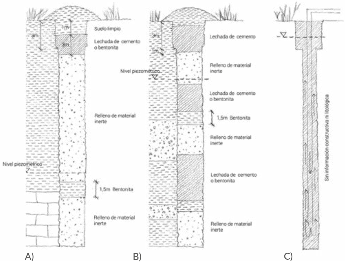
Figura 9.7. A) Alternativas de sellado en acuífero único, B) multicapa o C) sin información constructiva. (propio y modificado de ACA, 2009).
