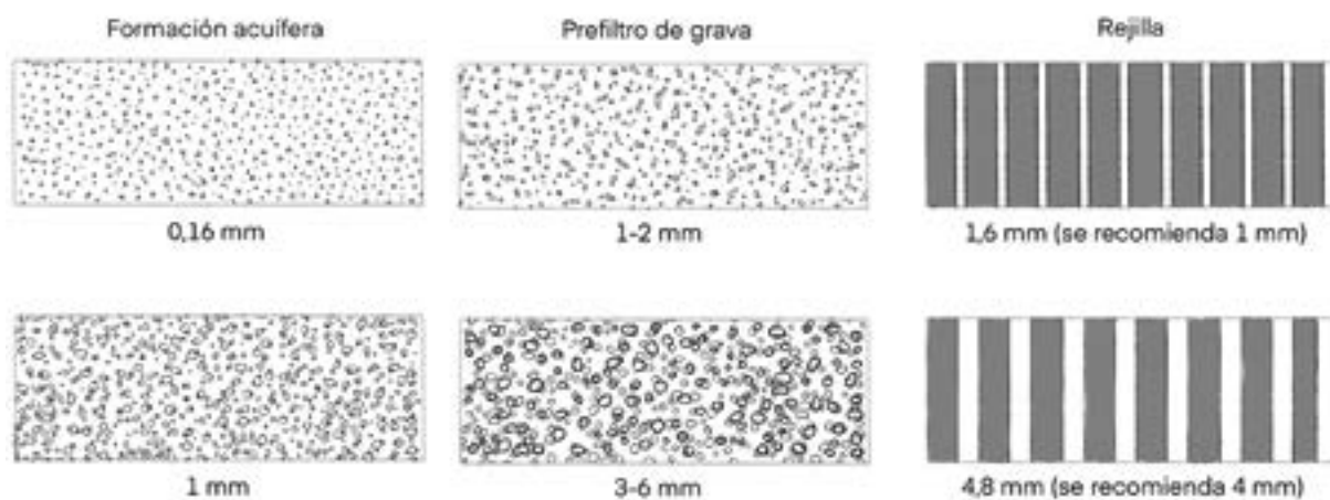
Figura 7.4.6. Relación entre el tamaño de grano de la formación acuífera a retener, el macizo de grava necesario y la apertura de rejilla adecuada.
