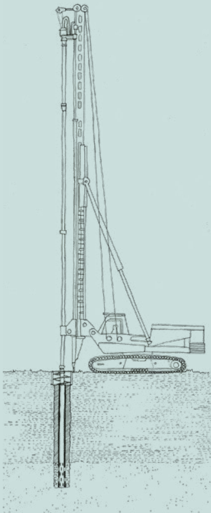
Figura 9.3. Operación de reperforación y destrucción de tubería.
