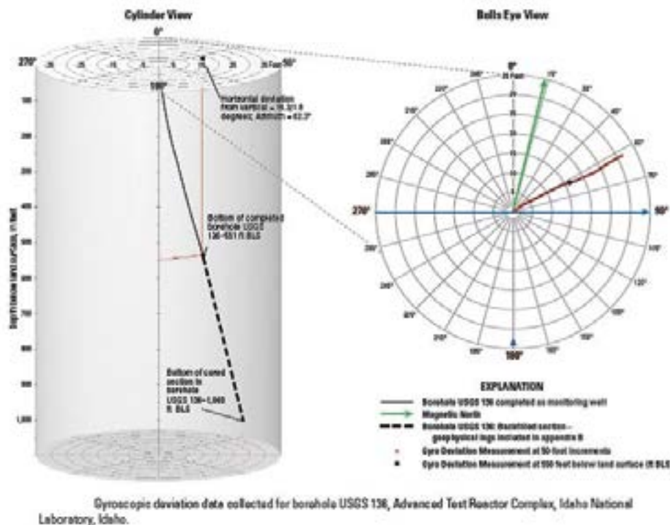
Figura 7.2.4. Ejemplo de diagráfias de verticalidad y desviación de un sondeo.
